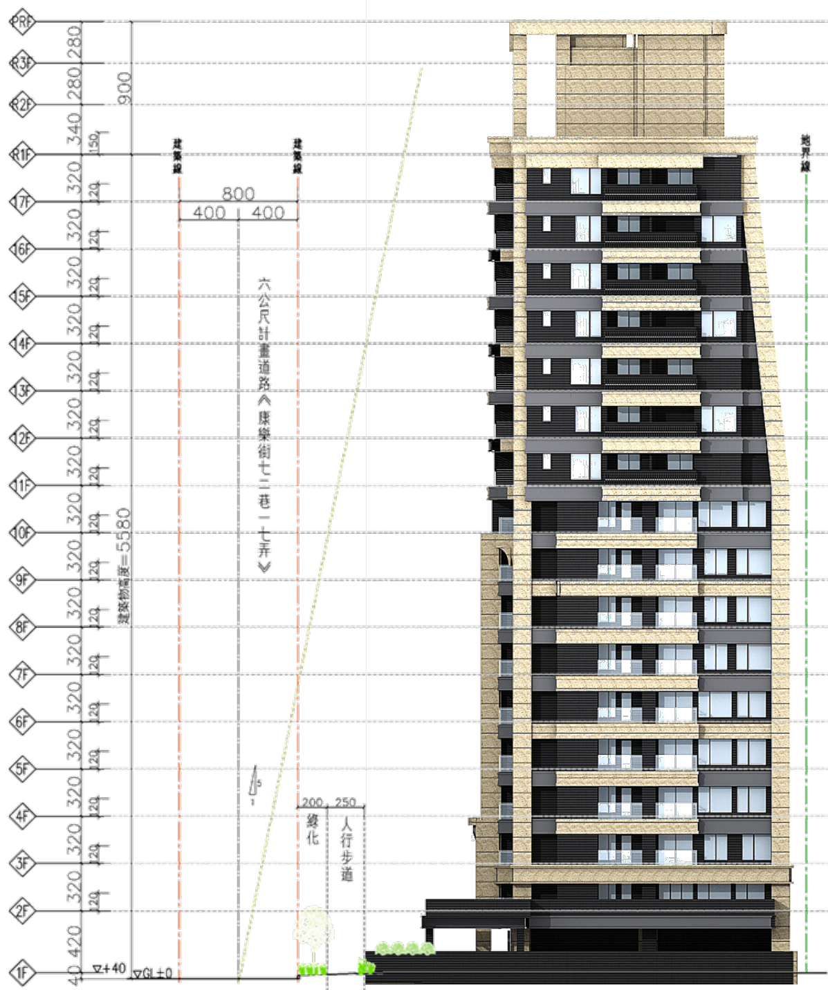
北向立面圖面圖
