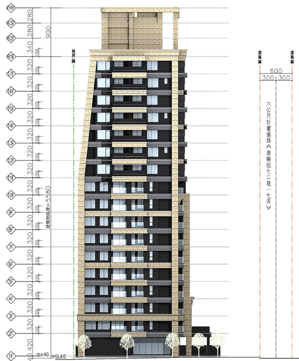
南向立面圖面圖
