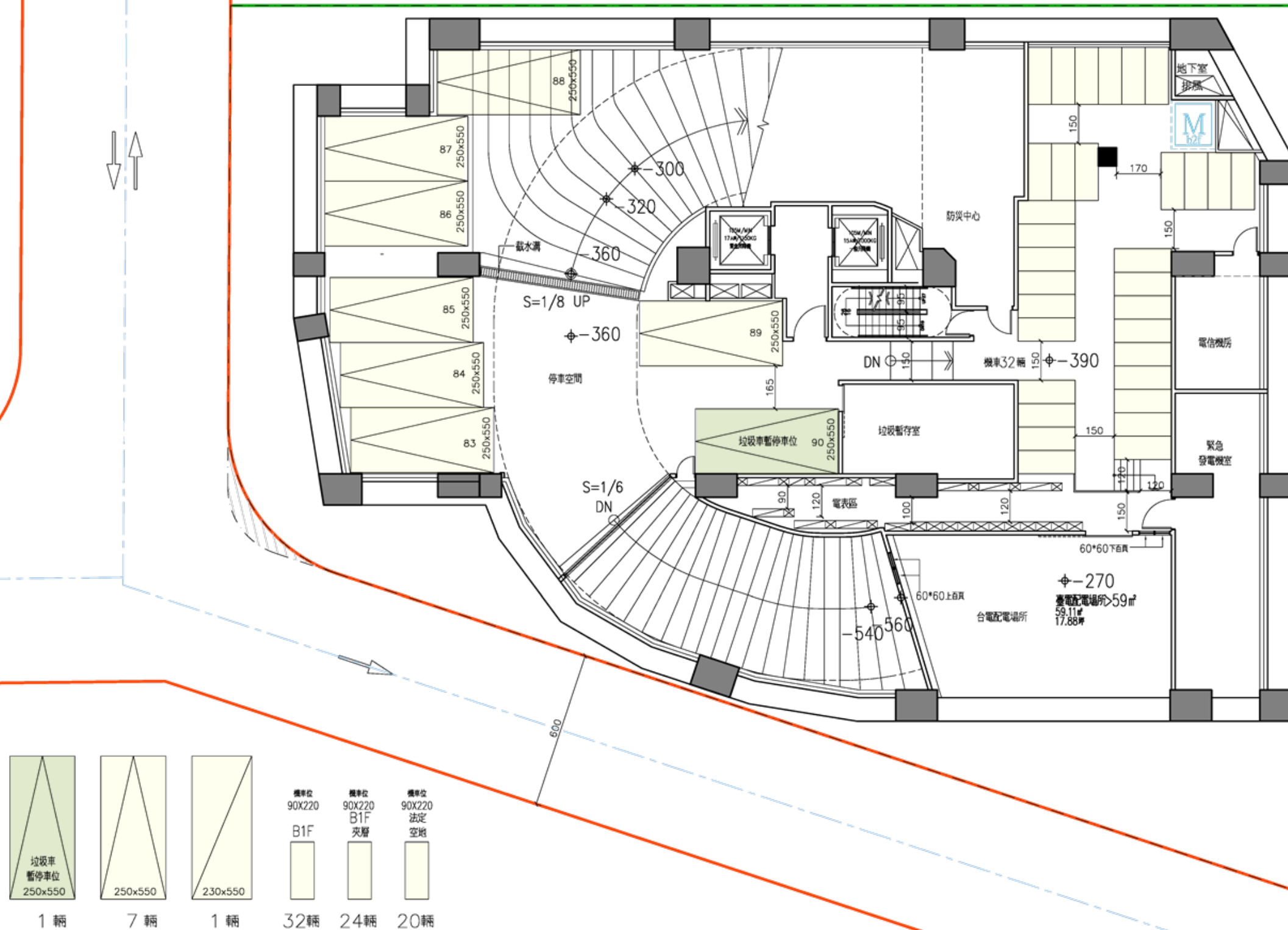
地下一層平面圖
