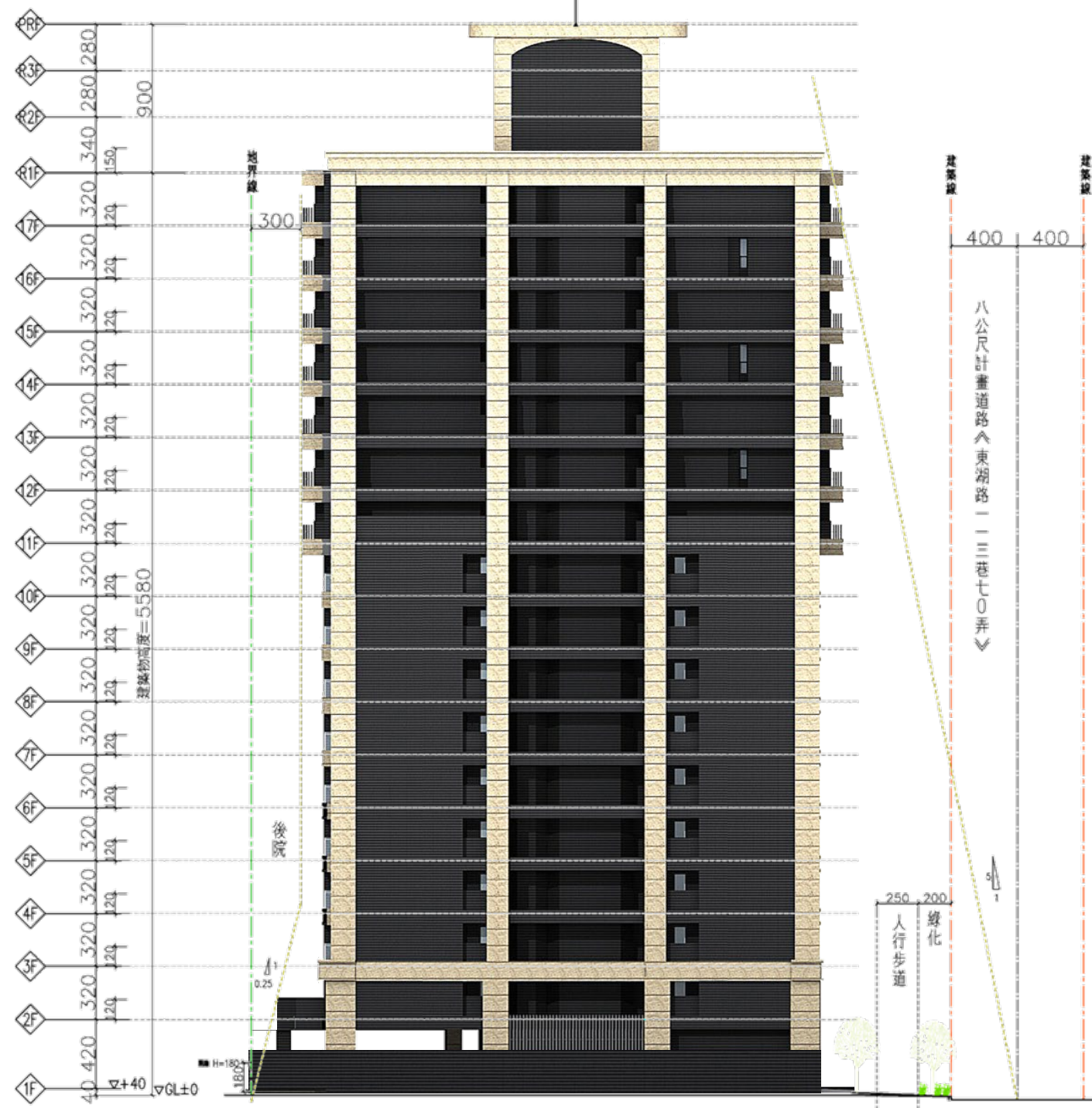
西向立面圖面圖
