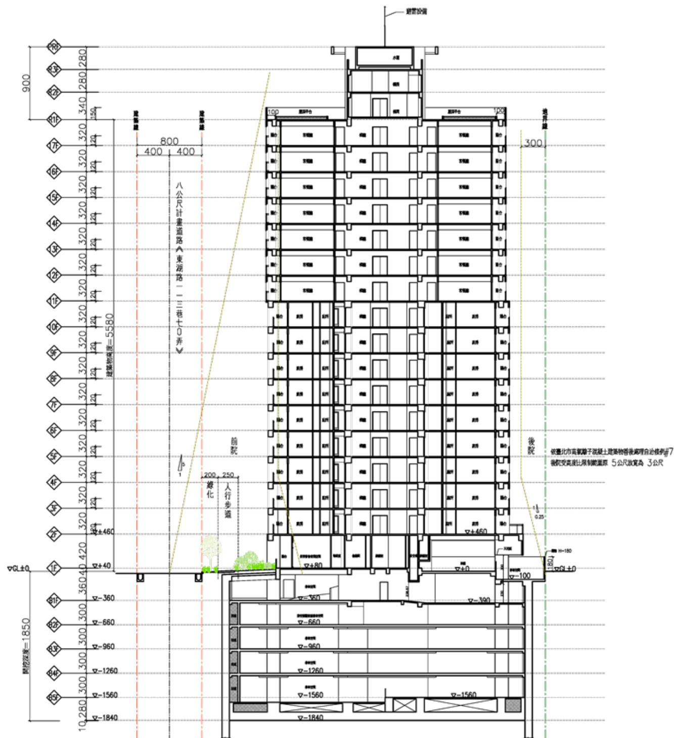
橫向剖面圖
