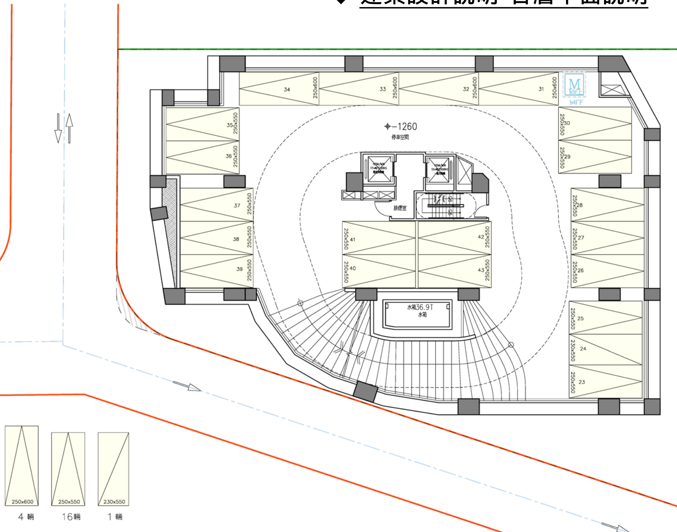
地下四層平面圖
